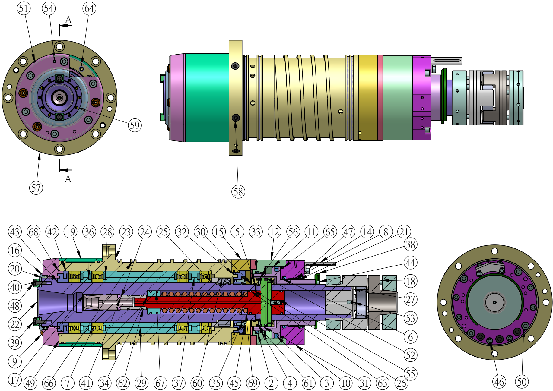
剖面圖 A-A
